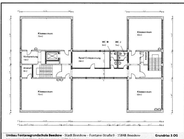
Umbau Fontanegrundschule Beeskow - Stadt Beeskow - Fontane-Straße9 - 15848 Beeskow Grundriss 3.0G
