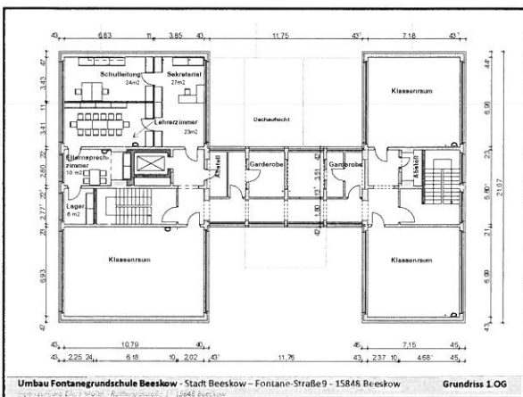
Umbau Fontanegrundschule Beeskow - Stadt Beeskow - Fontane-Straße9 - 15848 Beeskow Grundriss 1.0G
