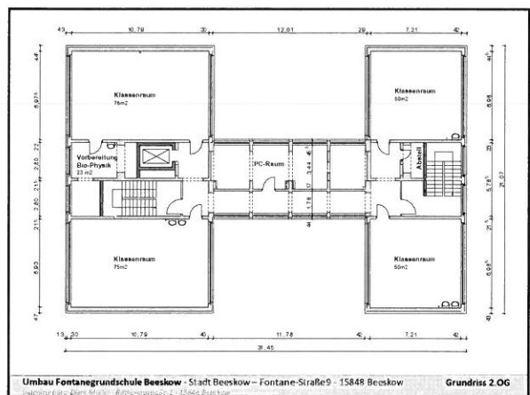
Umbau Fontanegrundschule Beeskow - Stadt Beeskow - Fontane-Straße9 - 15848 Beeskow Grundriss 2.0G
