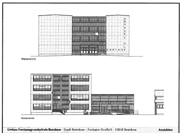
Umbau Fontanegrundschule Beeskow - Stadt Beeskow - Fontane-Straße9 - 15848 Beeskow Ansichten
