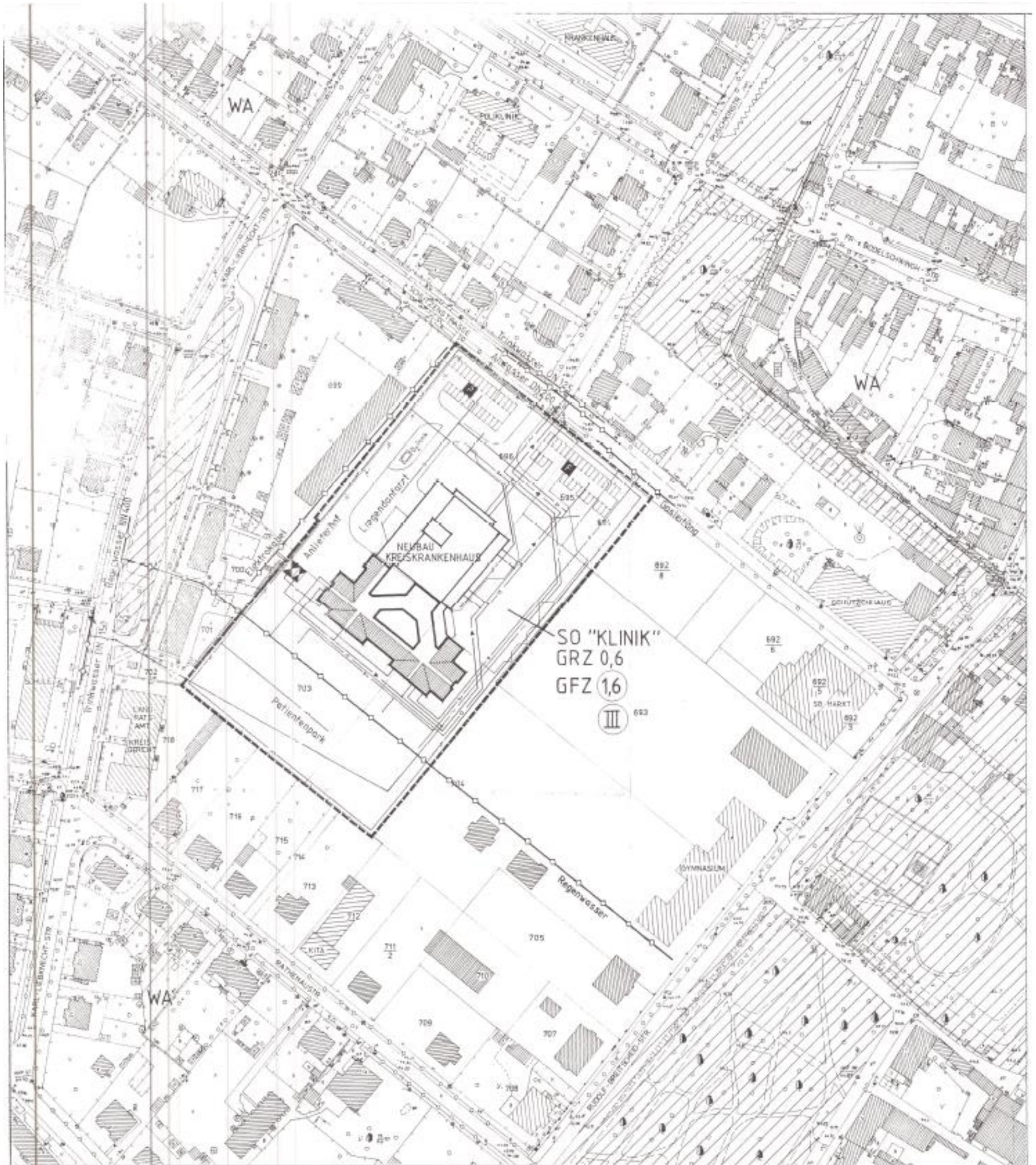
Auszug Planzeichnung zum Bebauungsplan Nr. S 1 „Kreiskrankenhaus Beeskow“
